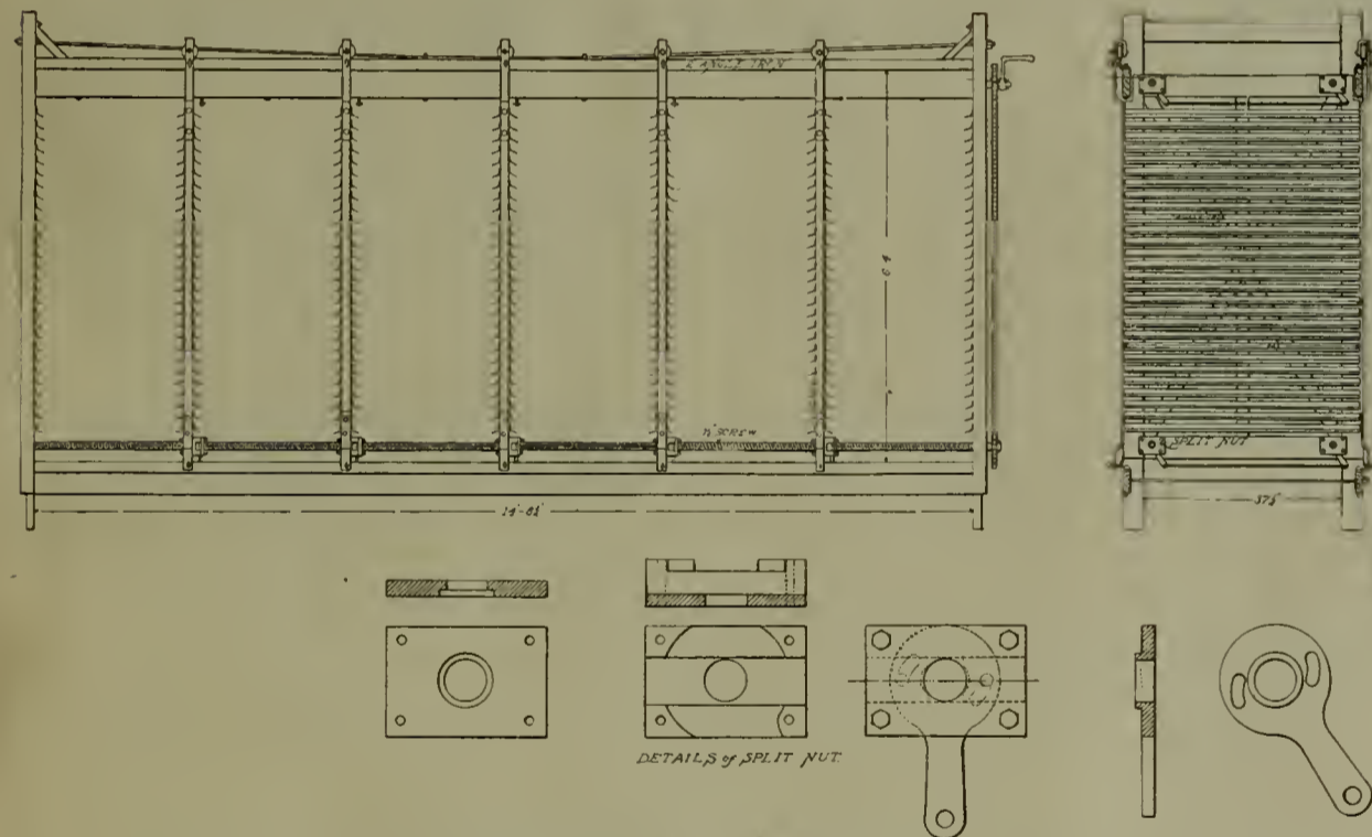
SASH RACK—L. S. & M. S. RY.
