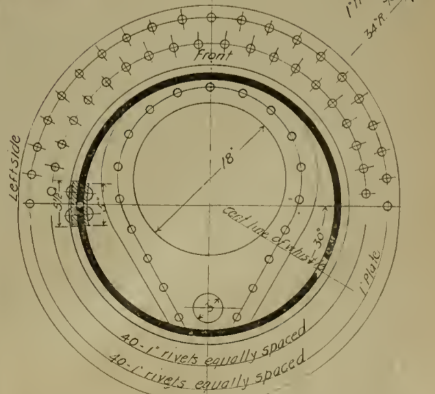
FIG. 3—DOME AND FASTENINGS A. T. & S. F. CONSOLIDATION.
