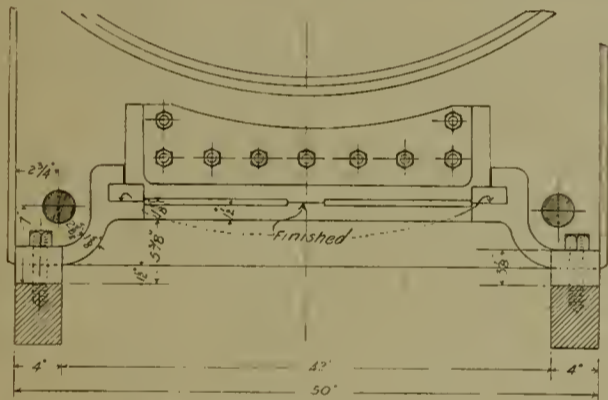
FIG. 5—FRAME BRACE, A. T. & S. F. CONSOLIDATION.
