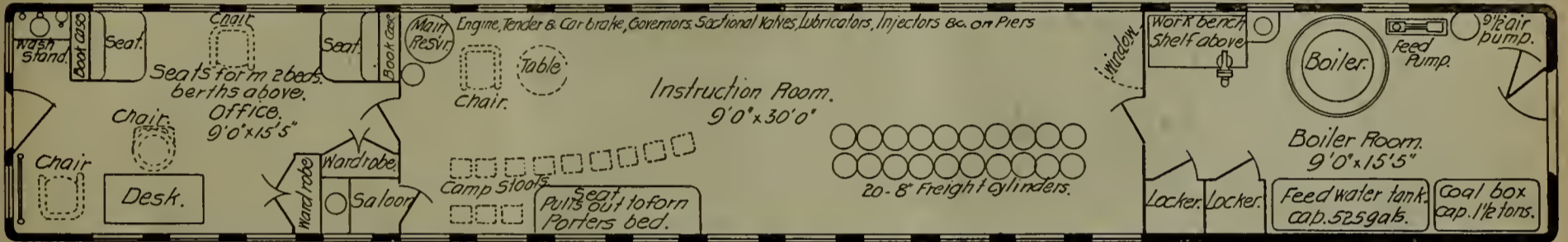
AIR BRAKE INSTRUCTION CAR—N. Y., N. H. & H. RY.—FLOOR PLAN.
