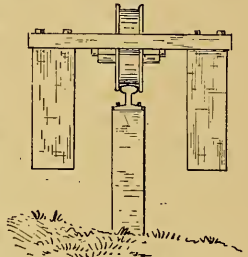
FIG. 6.—SERGEANT, 1825.
